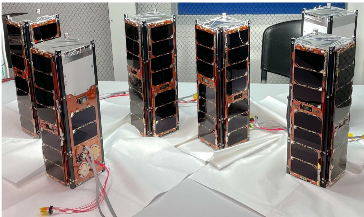
I 6 nanosatelliti H.E.R.M.E.S. in configurazione compatta (pannelli solari chiusi), al termine della loro integrazione presso la camera pulita di ASTRA Lab - Dipartimento di Scienze e Tecnologie Aerospaziali del Politecnico di Milano
